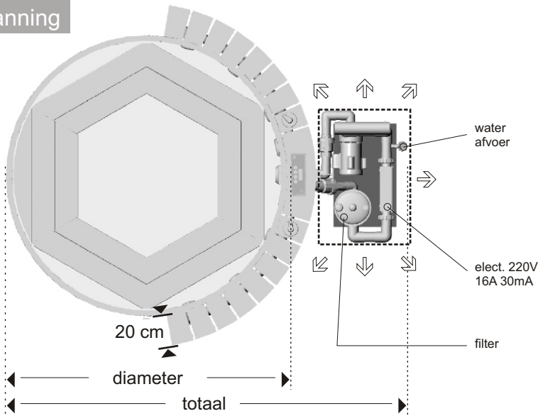
Afmetingen en inbouwmaten
